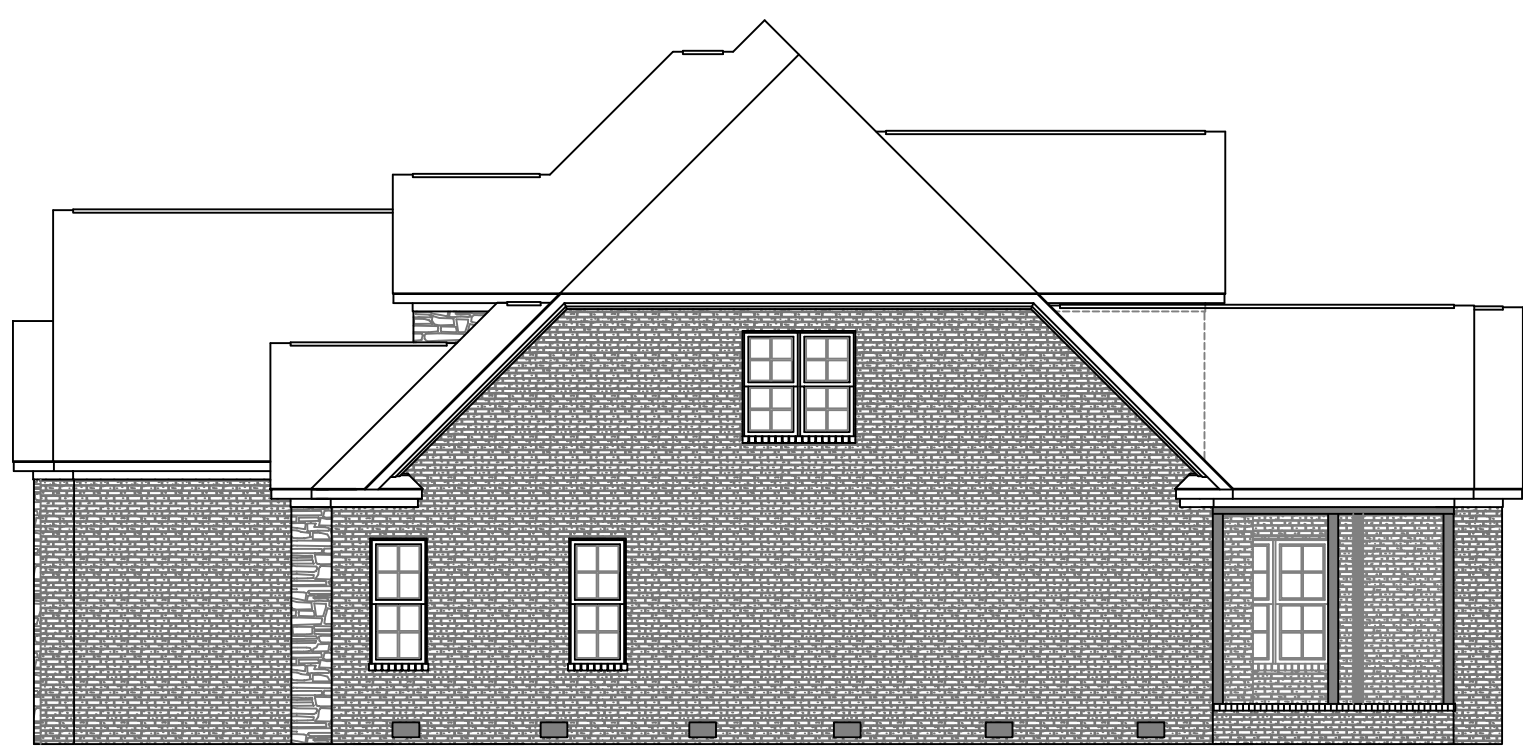
RIGHT ELEVATION
